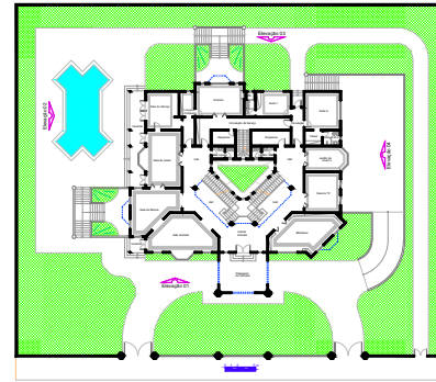
Térreo A = 567,71 m 2
